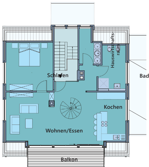
Obergeschoß
