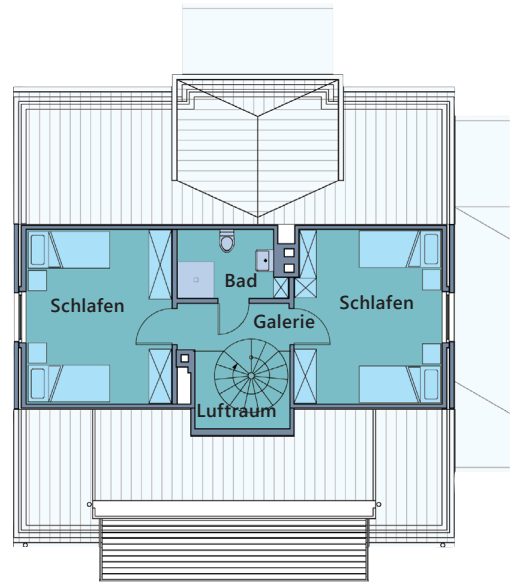
Dachgeschoß
